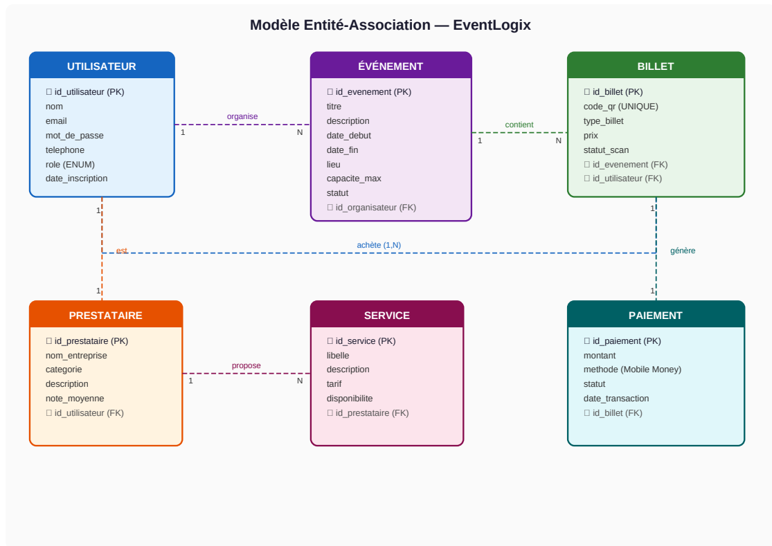
FIGURE 2.2 – Modèle Entité-Association — EventLogix
