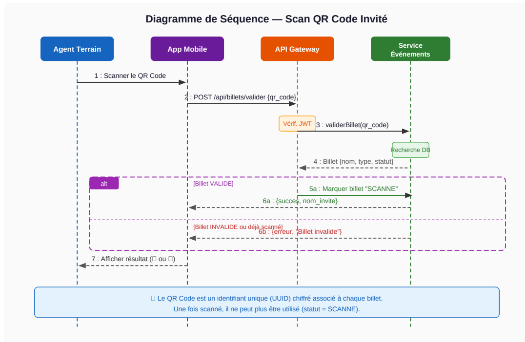
FIGURE 2.3 – Diagramme de séquence — Scan QR Code invité
