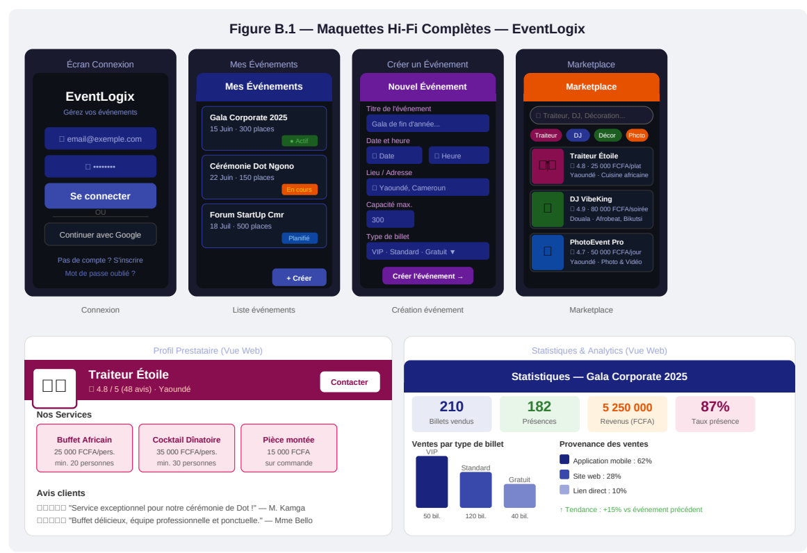
FIGURE B.1 – Maquettes Hi-Fi complètes — EventLogix
